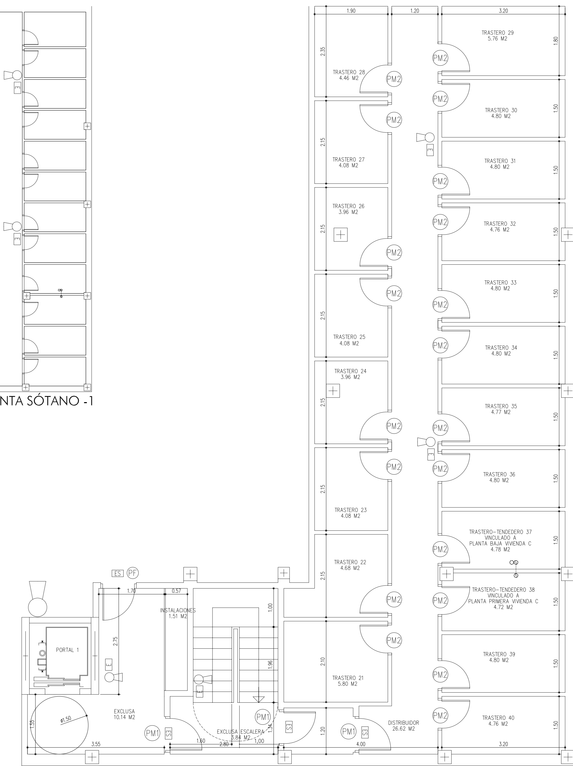
DETALLE DE TRASTEROS DE PORTAL 1 EN PLANTA SÓTANO -1 ESCALA 1/50
