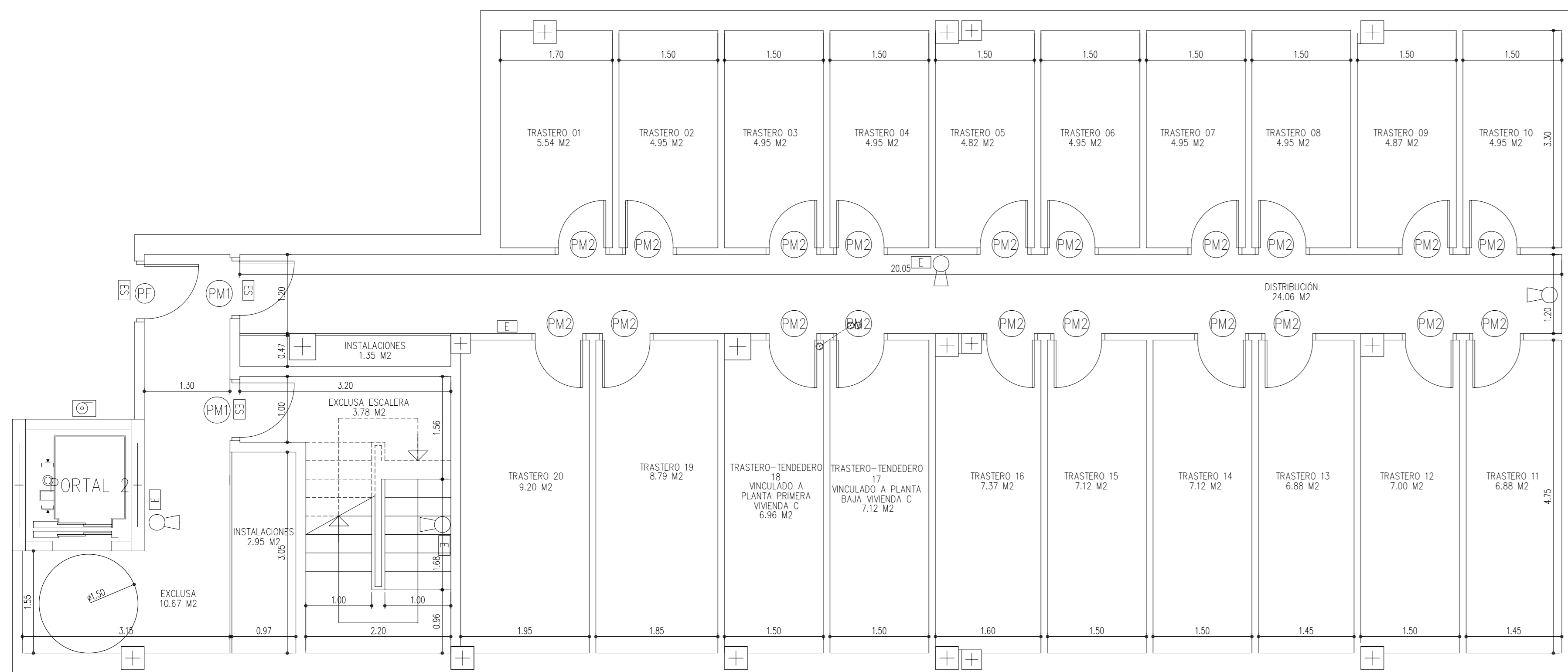
DETALLE DE TRASTEROS DE PORTAL 2 EN PLANTA SÓTANO -2 ESCALA 1/50
